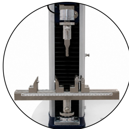
Mordazas de flexión de 3 puntos
