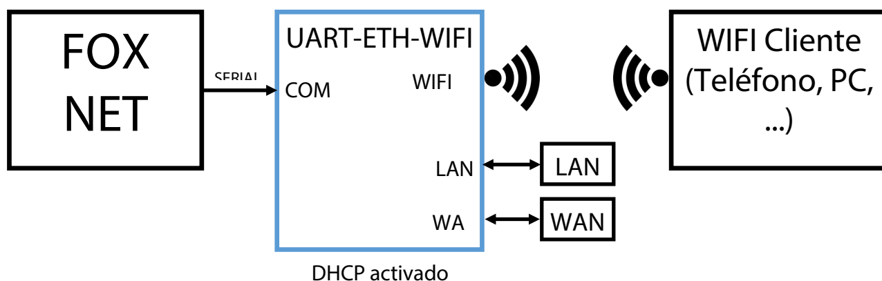
Imagen 4: Modelo default.
