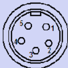
Conector redondo de 5 pines
